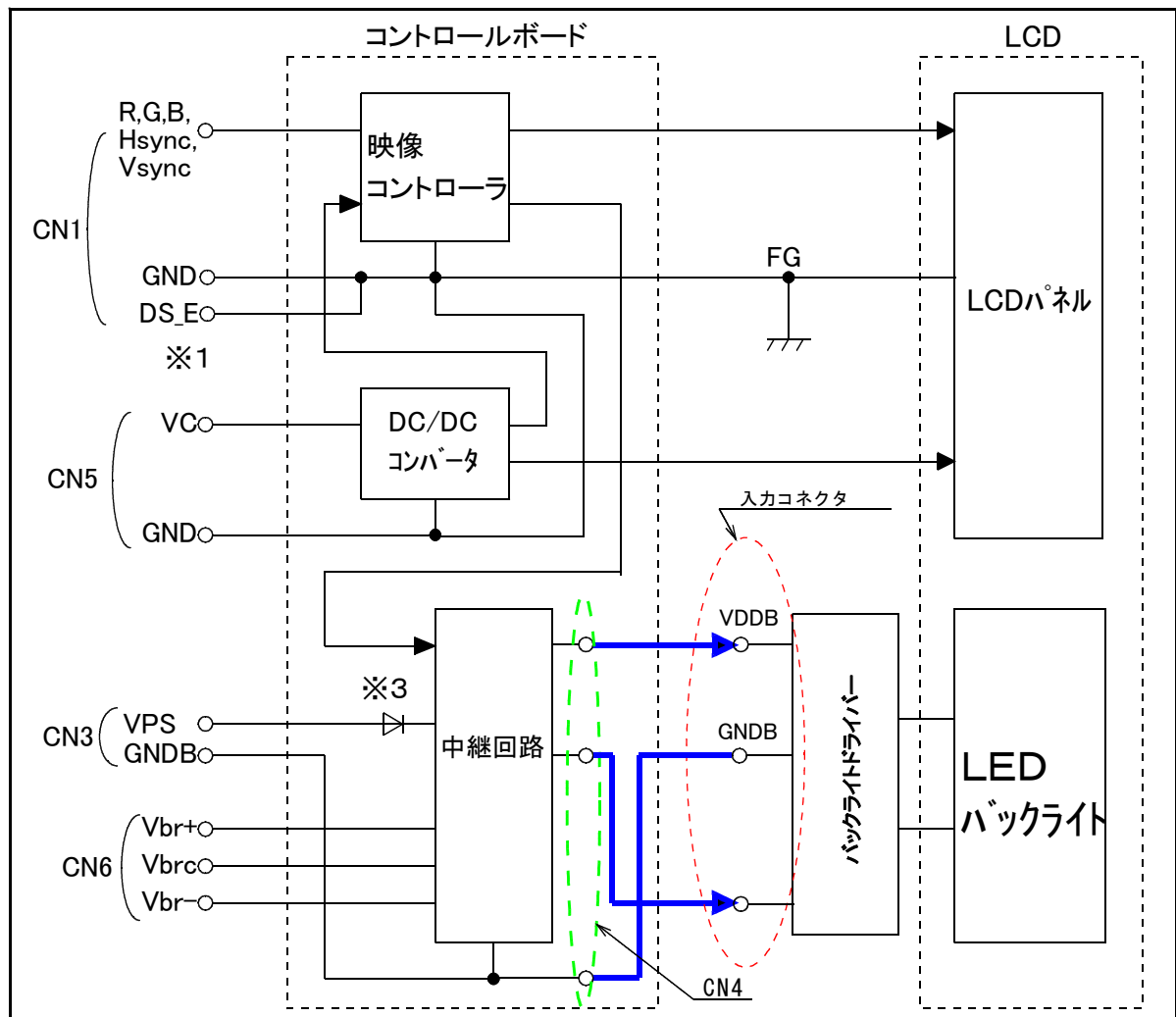
「ILB-6448V-104」ブロック図
